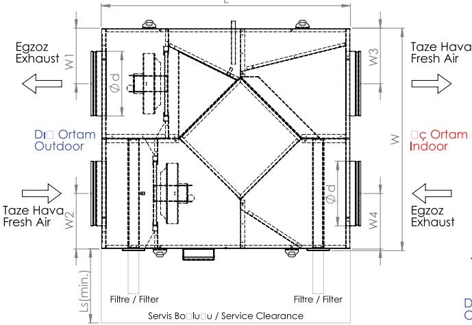
VHR 20/23
